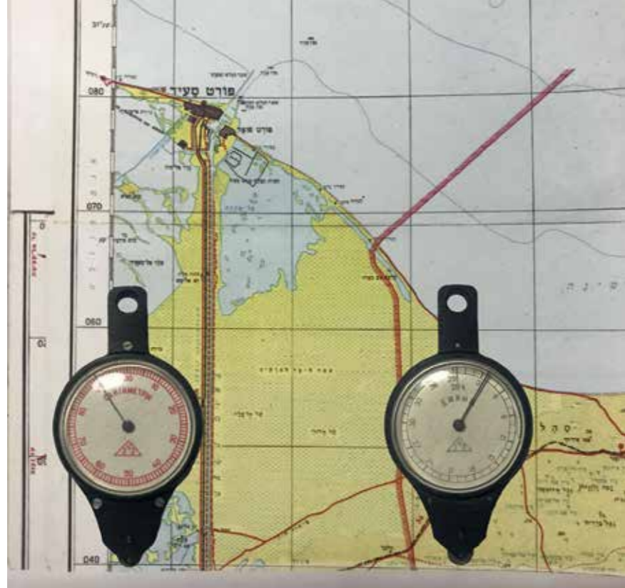
Курвиметр изготавливался на Златоустовском часовом заводе (ЗЧЗ)
